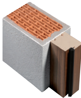
RAHMENSTOCK RSTA 75/66 in der Laibung montiert, auch in Verbindung mit Seitenteil- bzw. Oberlichte möglich
