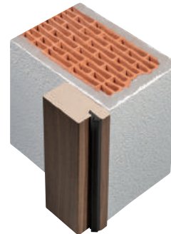
BLENDRAHMEN BM 45 vor der Laibung montiert, perfekte Lösung für Renovierer
