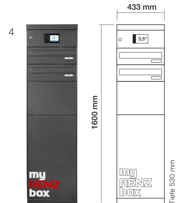
4 eQUBO, mit myRENZbox-Steuereinheit 3,5", zwei Briefkästen, einem Paketkasten M, einem Paketkasten XL gerades Dach Best.-Nr. 23-0-10034 schräges Dach Best.-Nr. 23-0-10035
