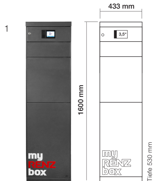
1 eQUBO, mit myRENZbox Steuereinheit 3,5", mit einem Paketkasten S, einem Paketkasten L, einem Paketkasten XL gerades Dach Best.-Nr. 23-0-10028 schräges Dach Best.-Nr. 23-0-10029
