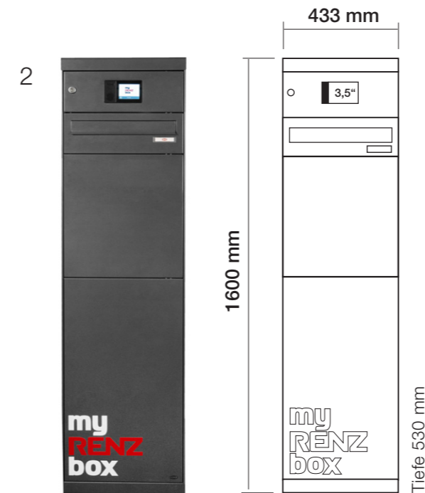
2 eQUBO, mit myRENZbox Steuereinheit 3,5", einem Briefkasten, einem Paketkasten L, einem Paketkasten XL gerades Dach Best.-Nr. 23-0-10032 schräges Dach Best.-Nr. 23-0-10033
