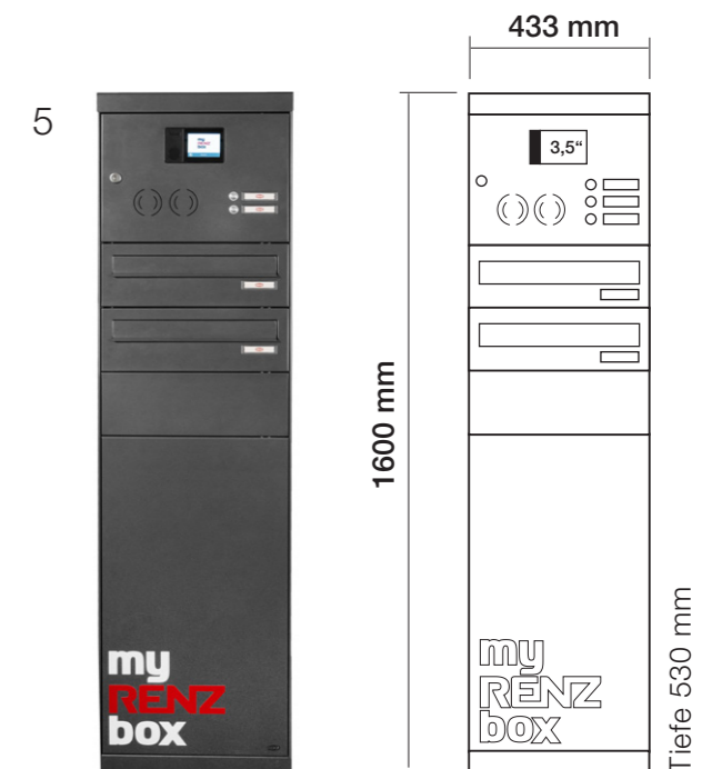
5 eQUBO, mit myRENZbox-Steuereinheit 3,5", zwei Briefkästen, Sprechfeld, Licht-/Klingeltaster, einem Paketkasten S, einem Paketkasten XL gerades Dach Best.-Nr. 23-0-10036 schräges Dach Best.-Nr. 23-0-10037
