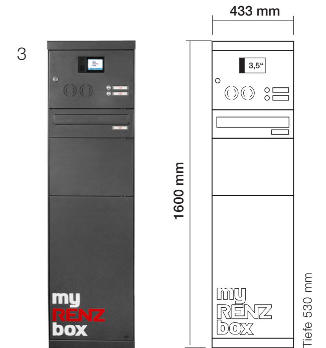
3 eQUBO, mit myRENZbox Steuereinheit 3,5", einem Briefkasten, Sprechfeld, Licht-/Klingeltaster, einem Paketkasten M, einem Paketkasten XL gerades Dach Best.-Nr. 23-0-10030 schräges Dach Best.-Nr. 23-0-10031
